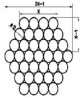
钢管捆总根数的计算示意图
