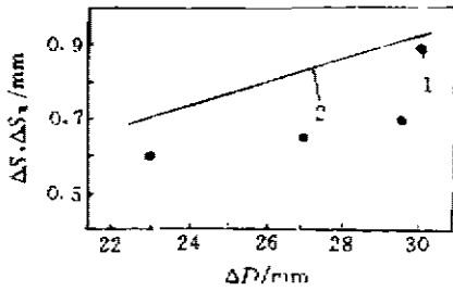
图3 Sc=7mm 系列
