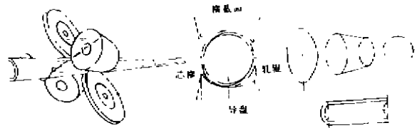
图1 Accu-Roll 轧管机
