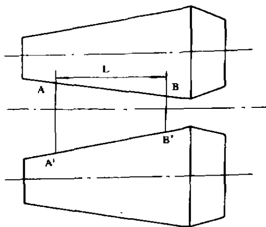
图 2 无辗轧角的 Accu Roll 轧管机孔型示意图。
