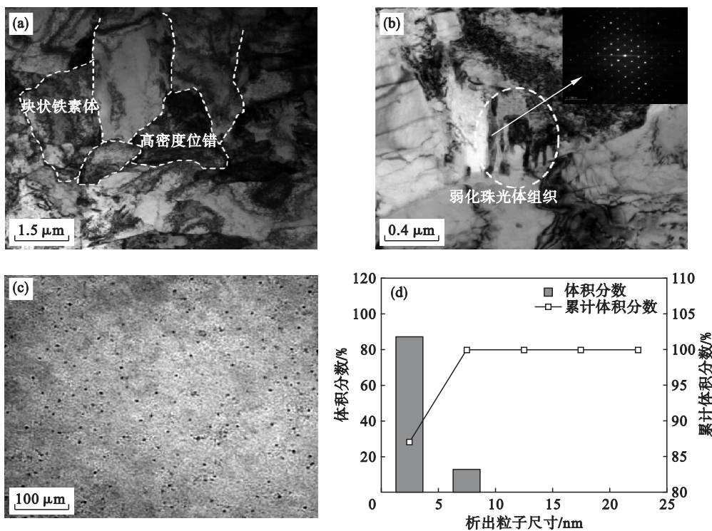
图4 实验钢 TEM 照片及纳米析出粒子尺寸统计
