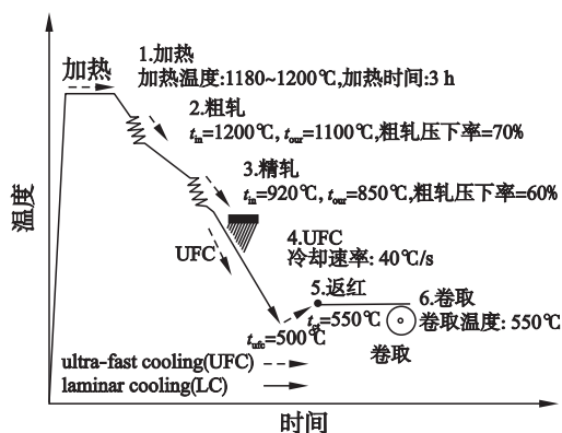
图1 实验钢控轧控冷工艺示意图
