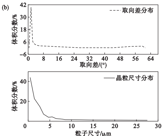
图 3 超快冷工艺下 X65 管线钢 EBSD 分析结果
