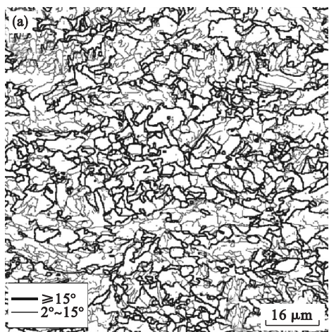
图 3 超快冷工艺下 X65 管线钢 EBSD 分析结果
