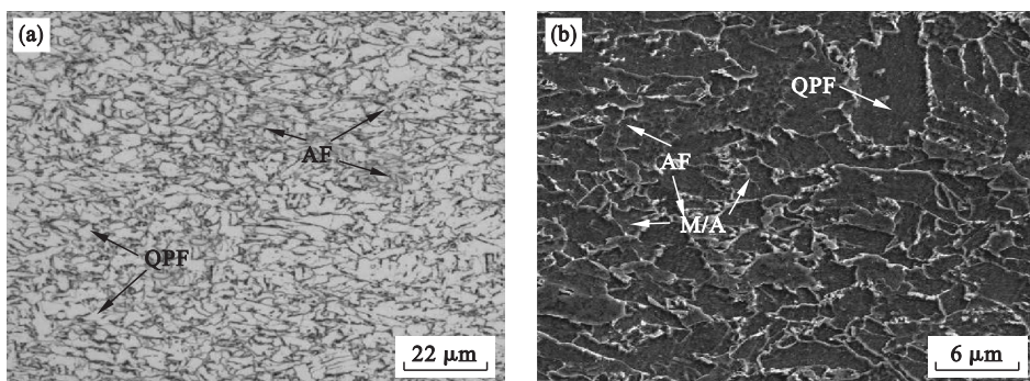
图 2 超快冷工艺下 X65 管线钢组织
